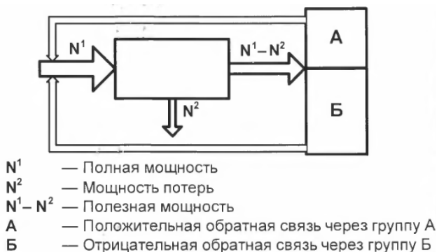
Рис. 4. Схема народного хозяйства как усилителя мощности
