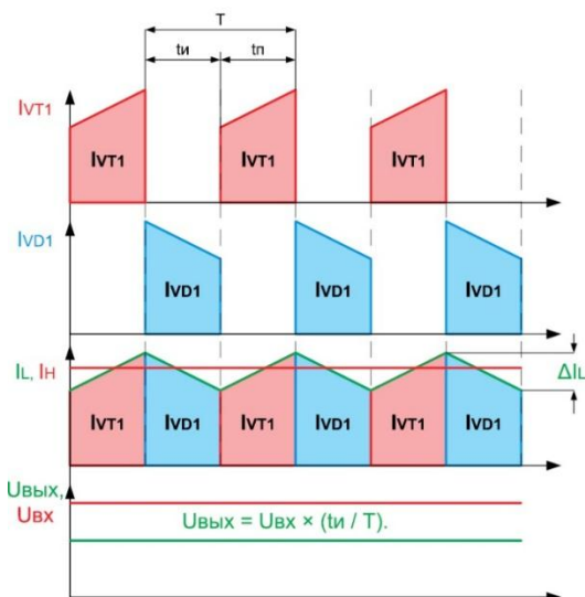
Рис. 3. Временные диаграммы напряжений и токов понижающего преобразователя
