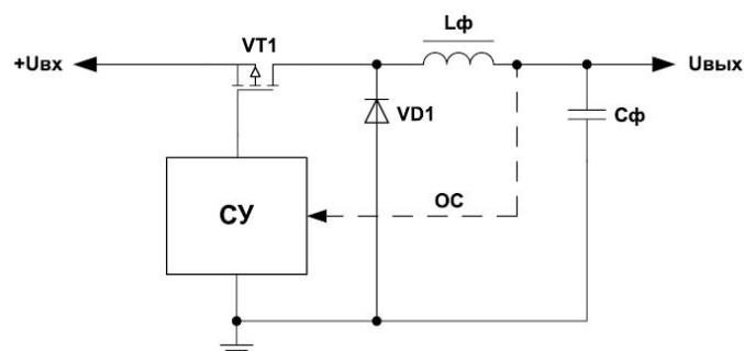
Рис. 1. Упрощенная схема понижающего преобразователя
