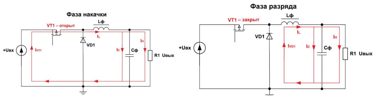
Рис. 2. Фазы работы понижающего преобразователя КС-01
